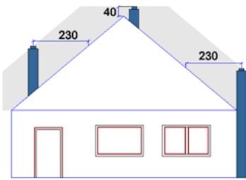
Ab 20° Dachneigung
