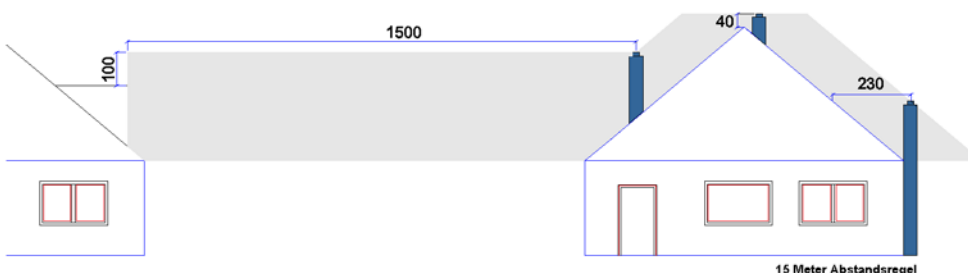
15 Meter Abstandsregel
