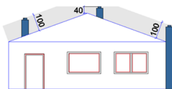
Bis 20° Dachneigung
